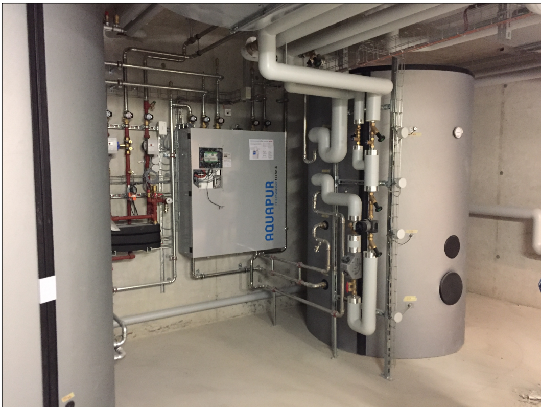
Blick in die Energiezentrale – oben die Heizwasseranschlüsse aus dem GBM-Wärmeverbund... ... unten einer der 3 Warmwassertanks für das auf dem Energiedach produzierte Duschwasser
