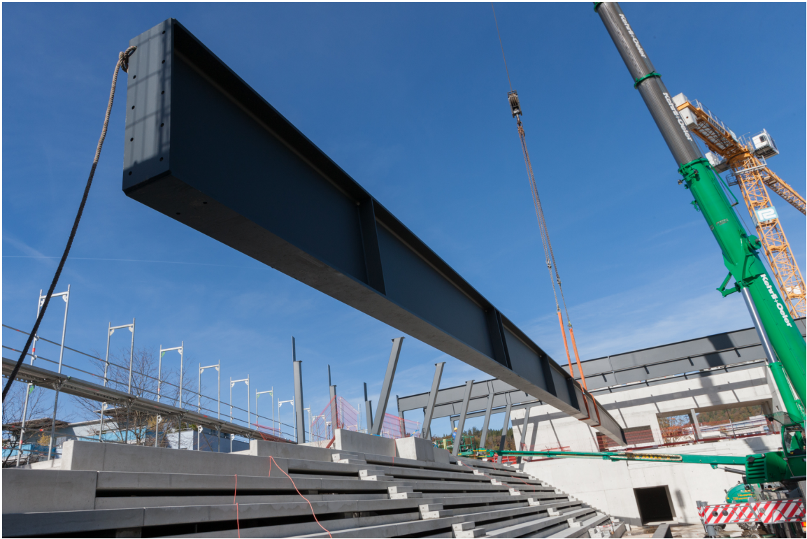
Impressionen von der Montage der Stahlkonstruktion des Hallendachs
