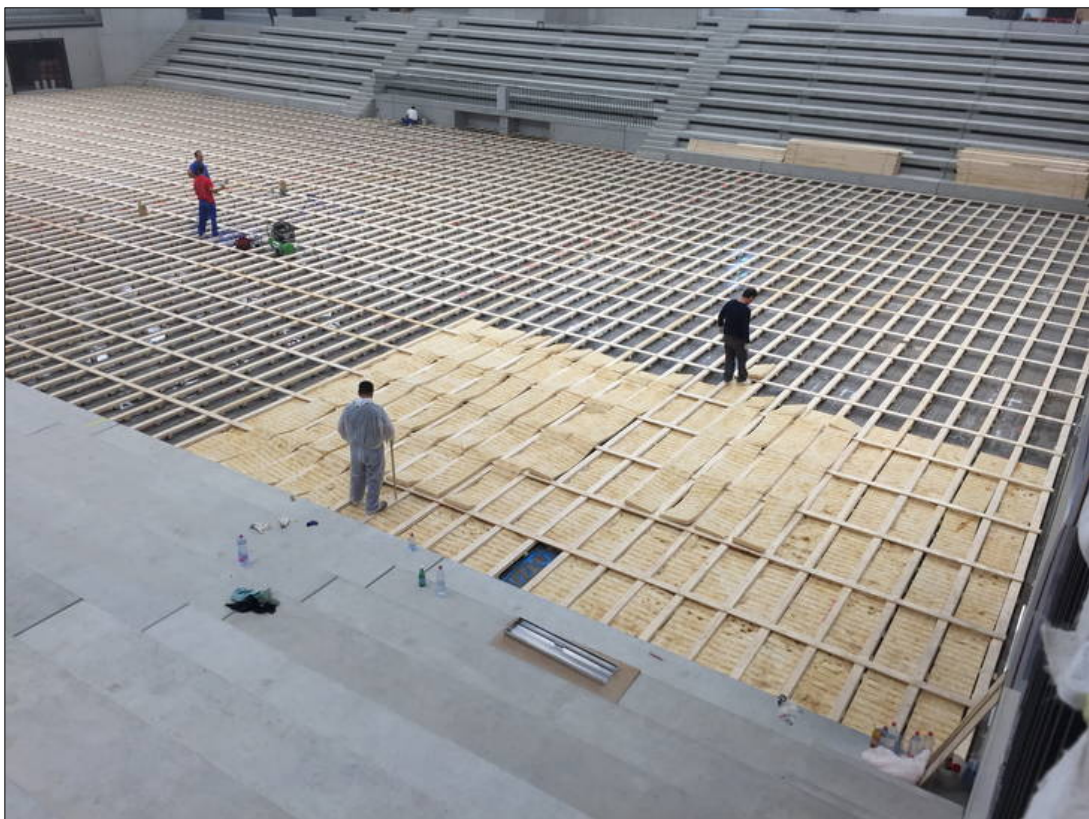
Als nächstes wurden Isoliermatten zwischen die ausnivellierten Latten gelegt ...
